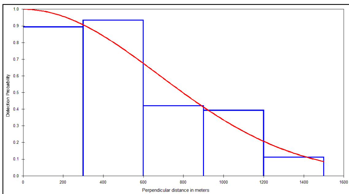
Figure 19 : Fonction de détection g correspondant à la détectabilité des groupes de Ziphii dans nos conditions d'observation (légende : en abscisse, la distance perpendiculaire x ; en ordonnée, la probabilité de détection g(x) non corrigée ; l'histogramme bleu correspond à nos données de terrain ; la courbe rouge représente la fonction g et est fournie par DISTANCE )
