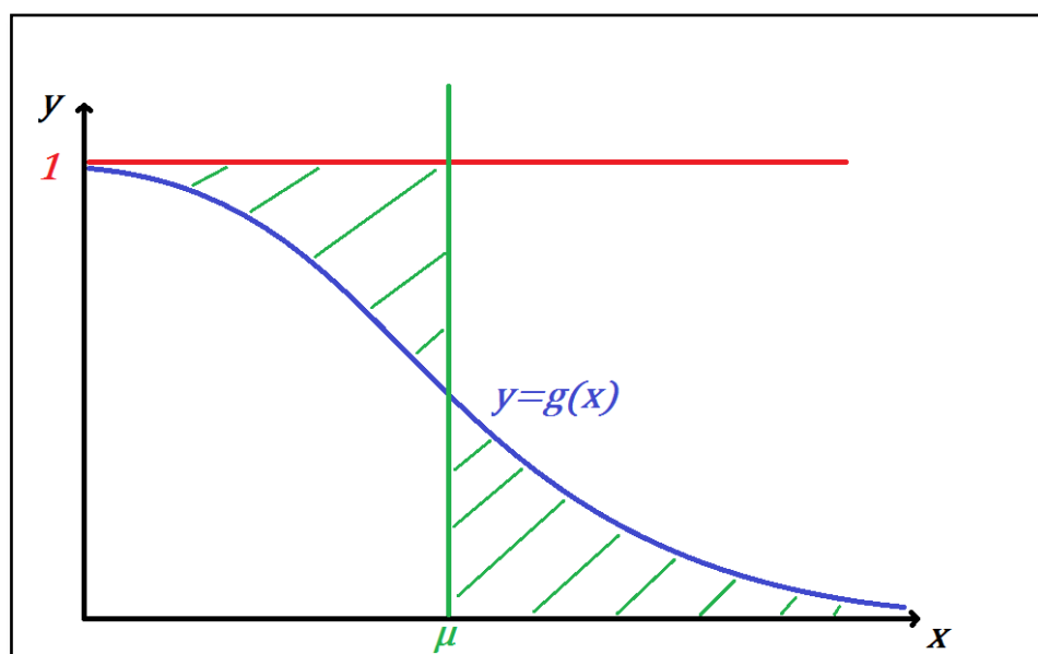
Figure 18 : Illustration de la définition de la demi-largeur effective de la bande d'échantillonnage \mu ; les deux zones hachurées en vert ont la même aire
